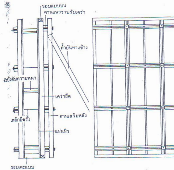
รูปแสดง ชิ้นส่วนประกอบของแบบหล่อกำแพง
